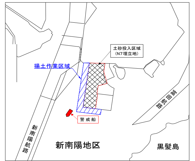
揚土場所詳細図(新南陽地区)
