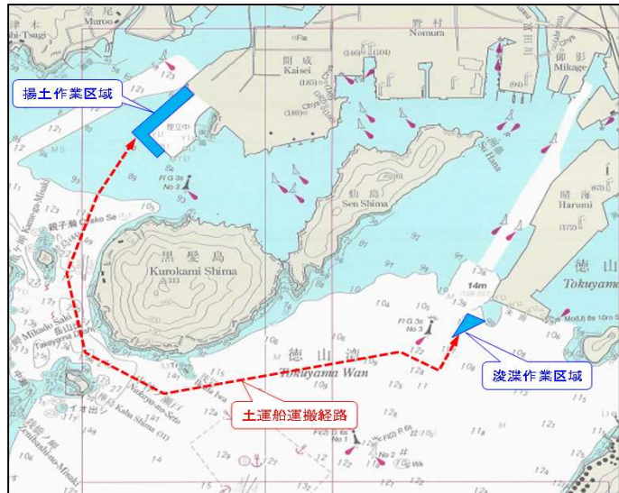
航路近傍作業図
