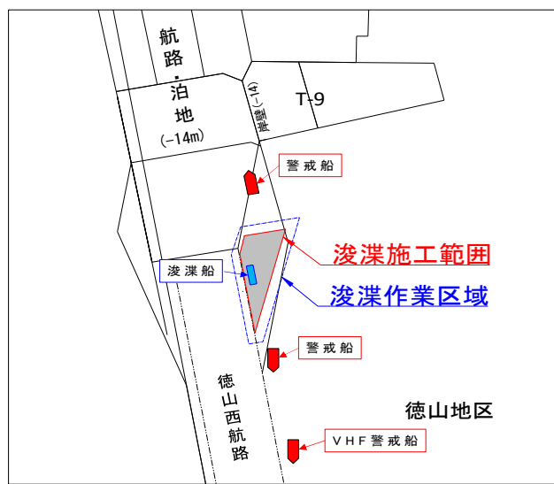
浚渫場所詳細図(徳山地区)
